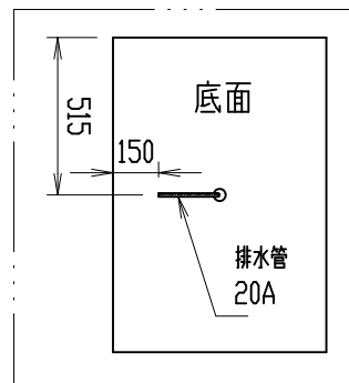
A矢視
